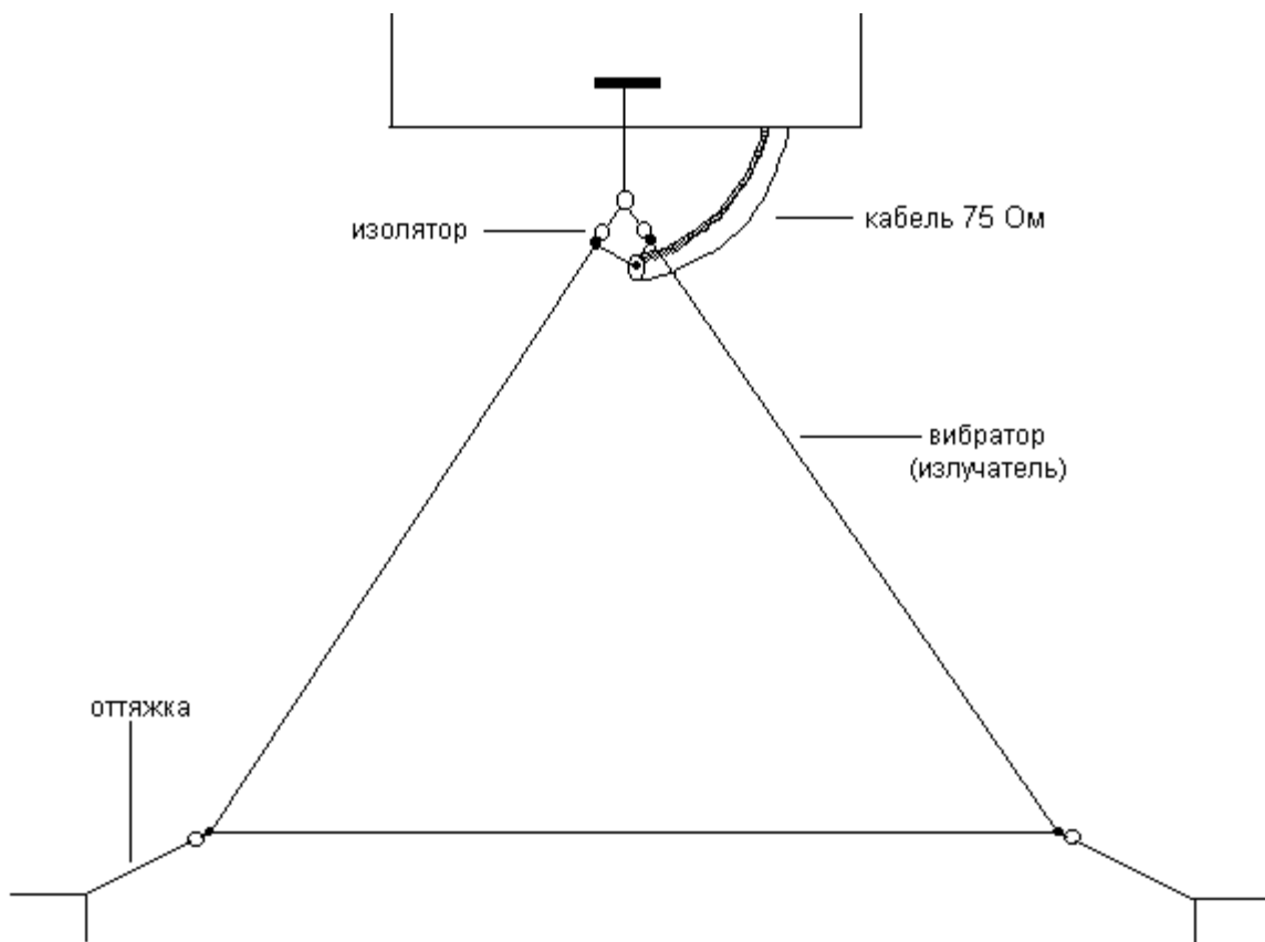
Рис. 2.12. Антенна «треугольник»
