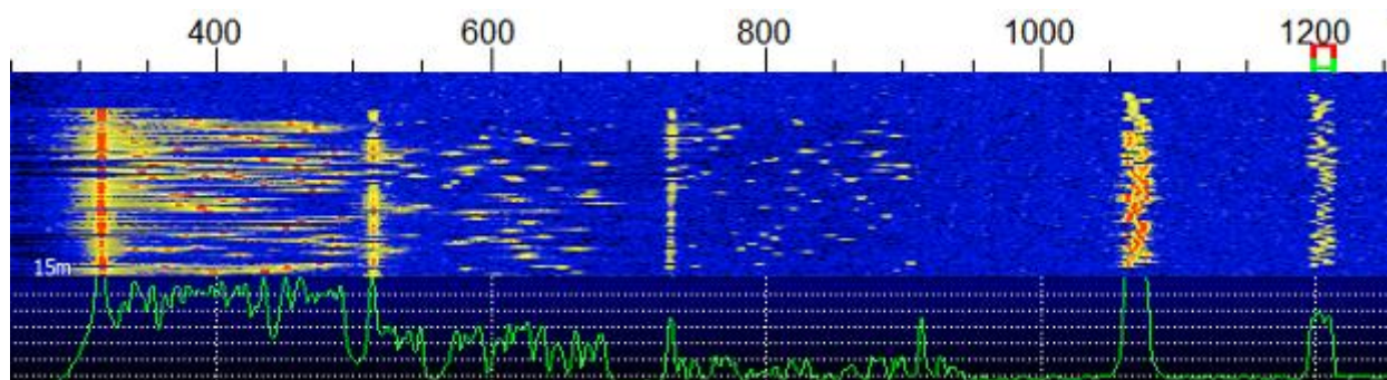
Рис.9.5. Вид сигналов JT65A (три слева) и JT9 (два справа), принятых с использованием программы WSJT-X
