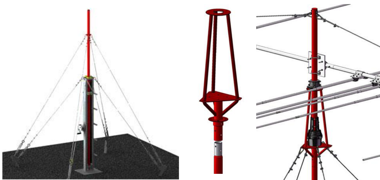
Рис. 2.9. Трубчатая мачта со станком-подъёмником СТ-S1Т
