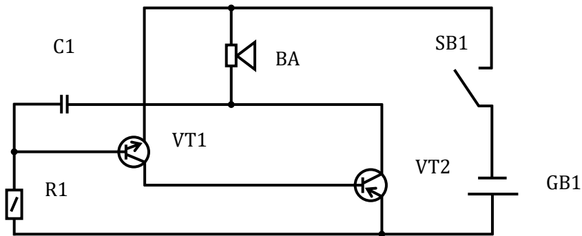
Рис. 8.3. Схема звукового генератора
