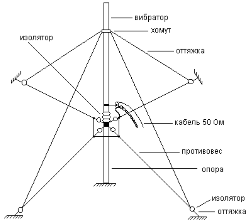
Рис. 2.13. Антенна «граунд-плэйн»
