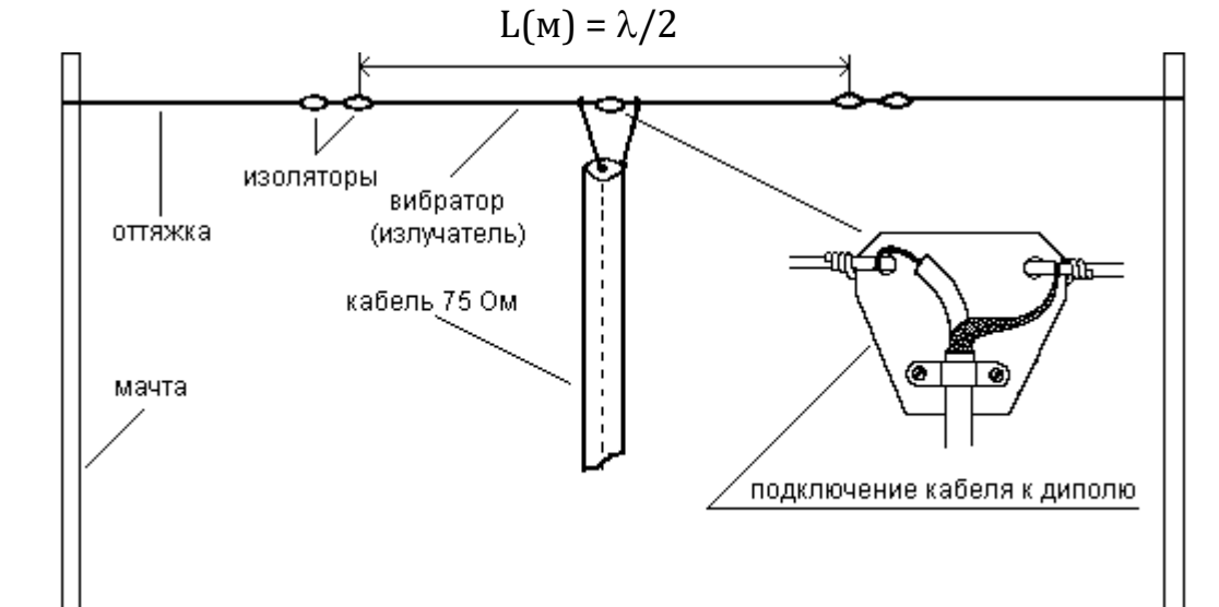
Рис .2.10. Антенна «диполь»
