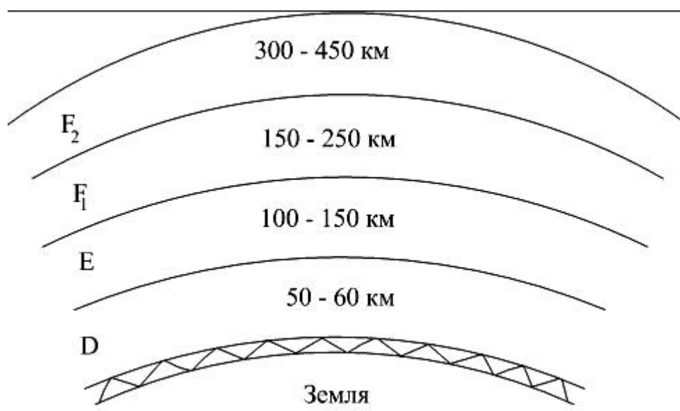
Рис. 2.2. Ионосферные слои
