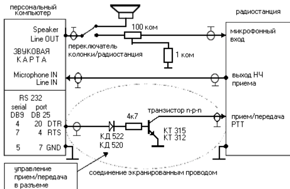
Рис. 9.1. Подключение «компьютер-трансивер»
