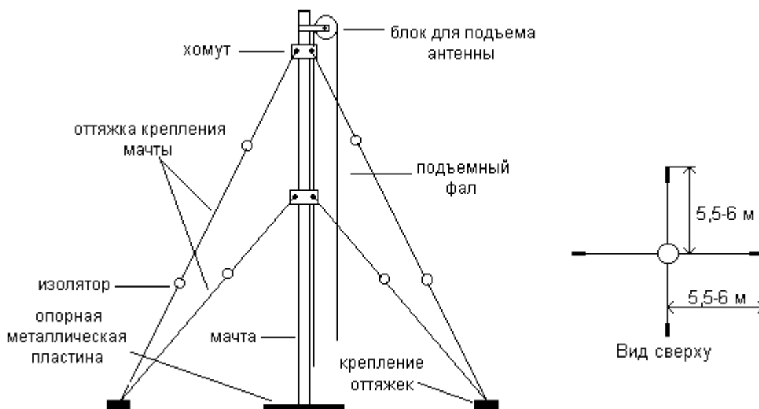
Рис. 2.8. Антенная мачта в развернутом виде
