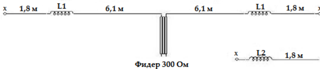
Рис. 2.14. Антенна «укороченный диполь»
